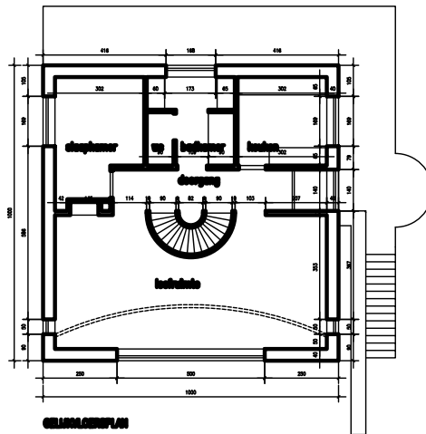
KESİM PLANI
